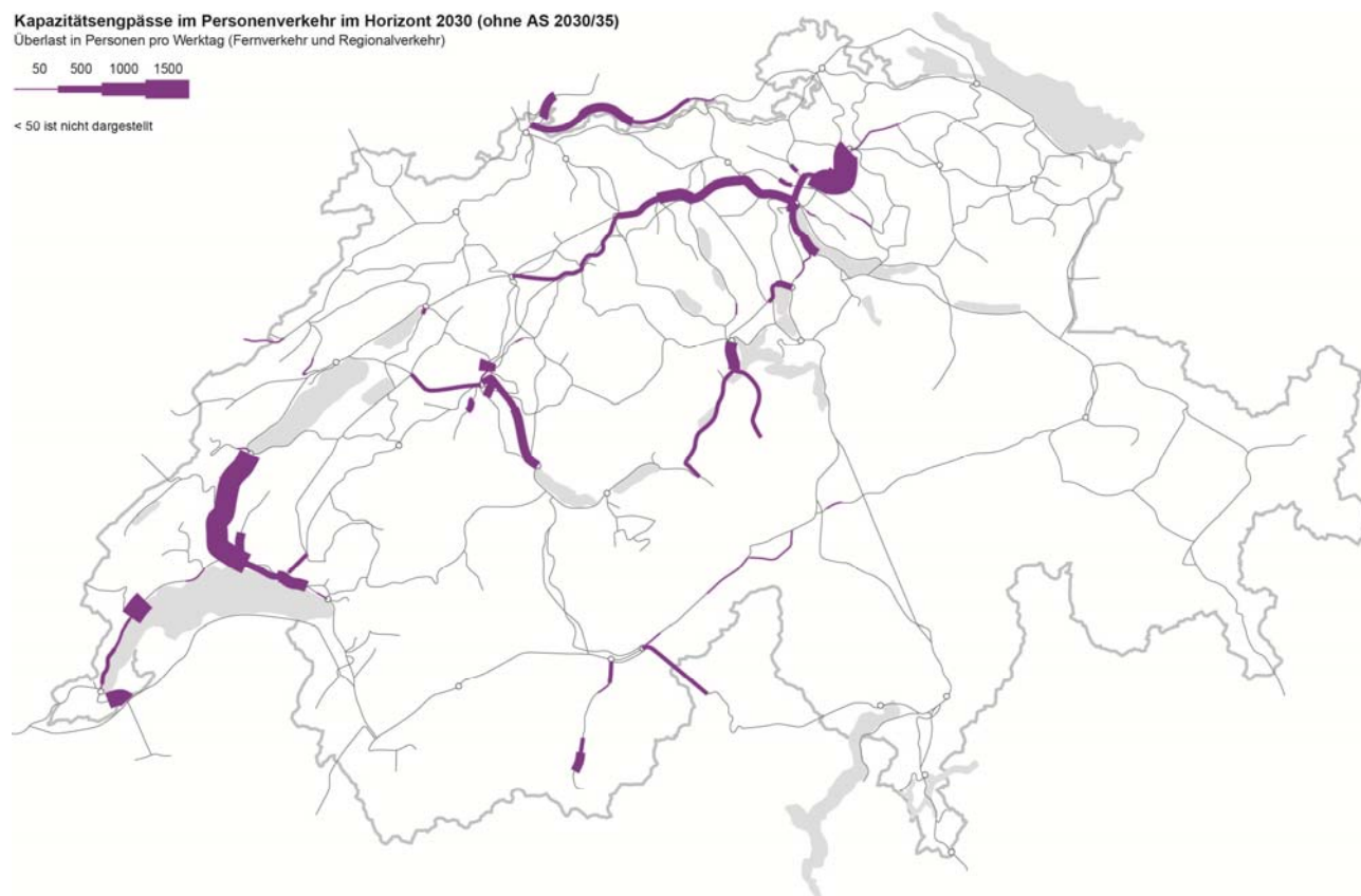
Abbildung 5: Bedarfsanalyse Personenverkehr: Kapazitätsengpässe im Personenverkehr im Horizont 2030 (ohne Ausbauschritt 2030/35)
